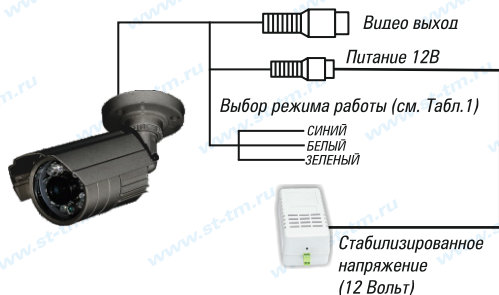
Рис.1 Схема подключения
