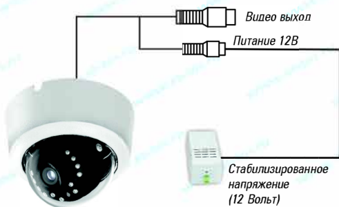
Рис.1 Схема подключения
